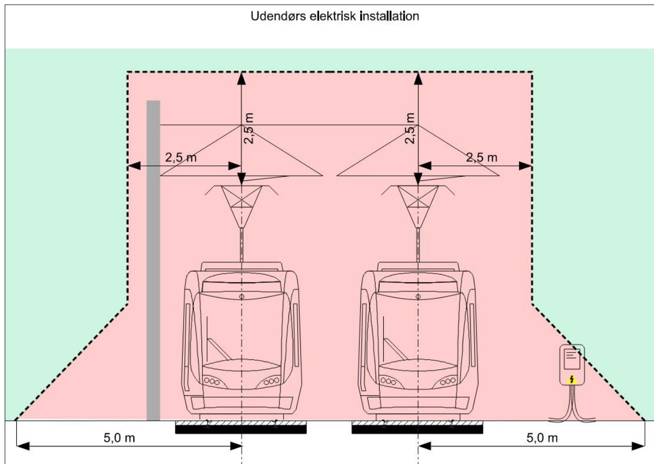
Principskitse
