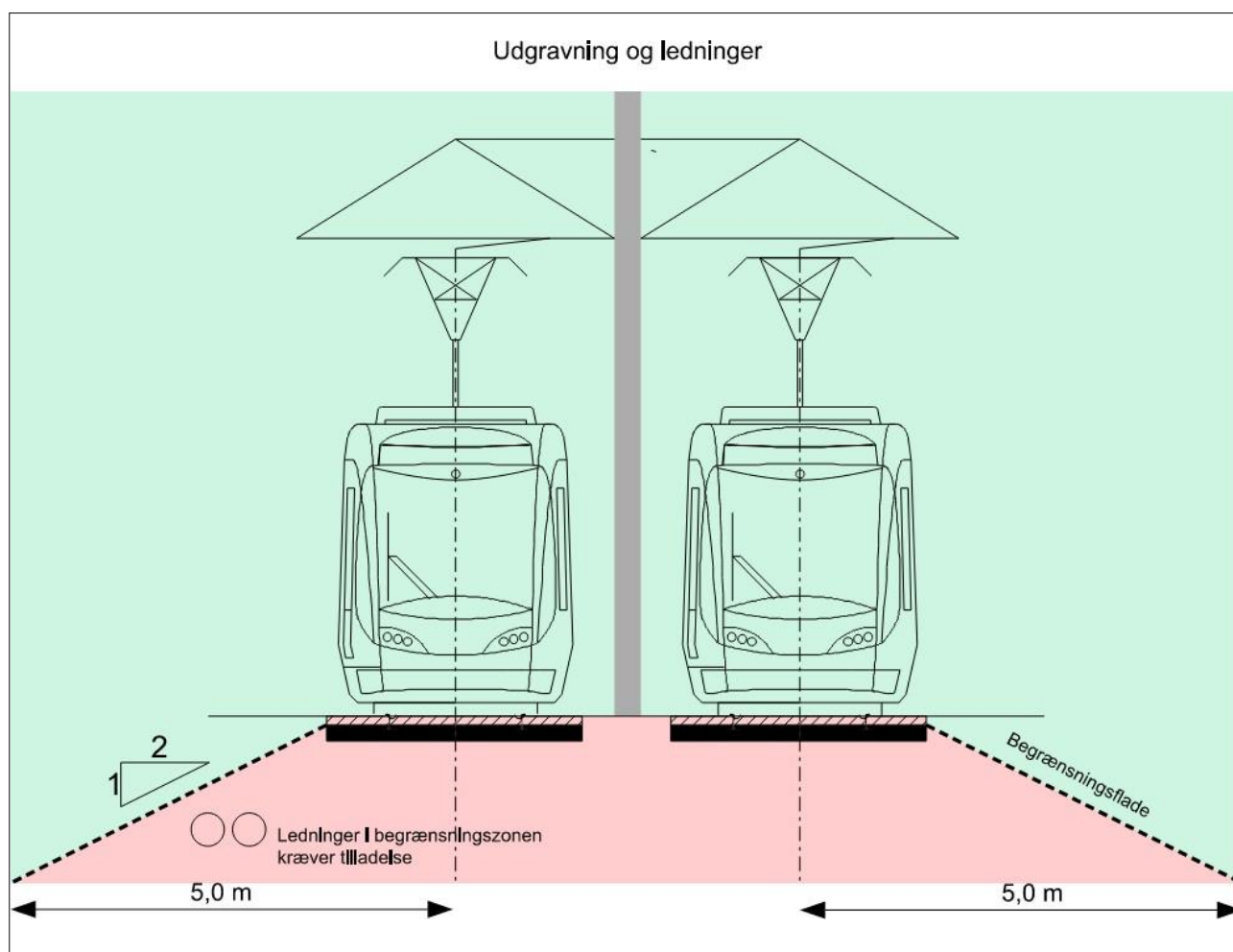
Principskitse
