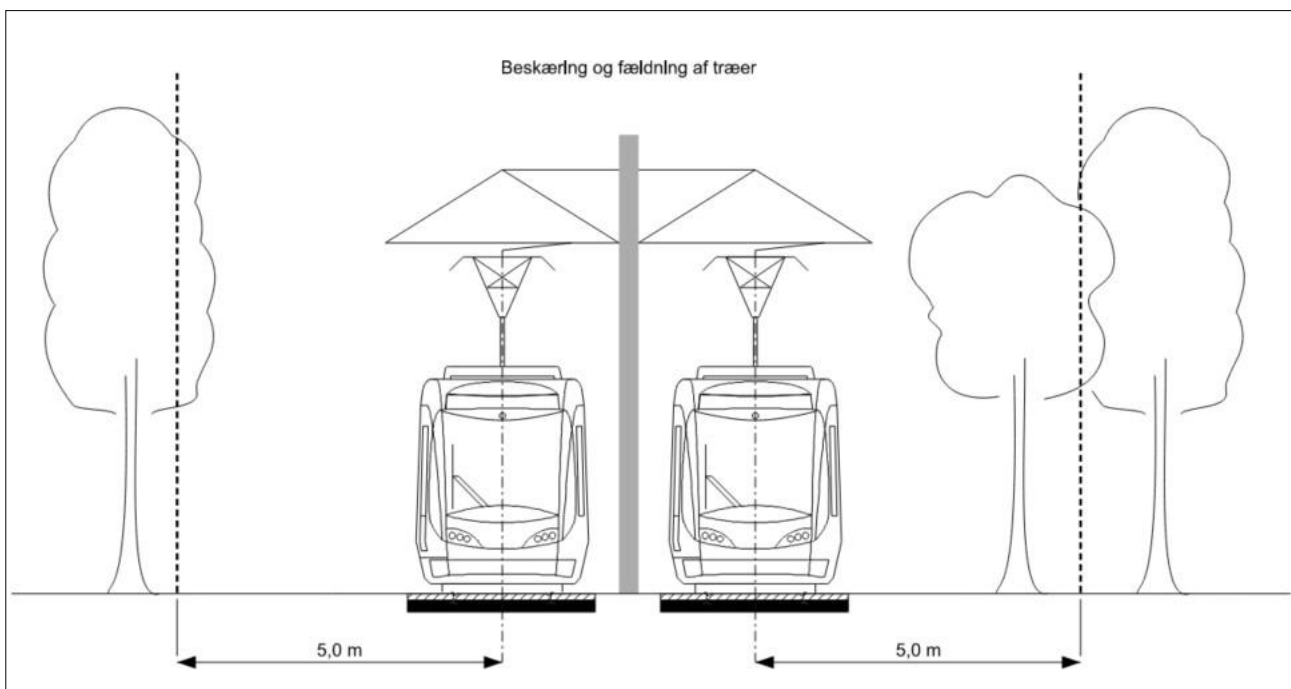
Principskitse
