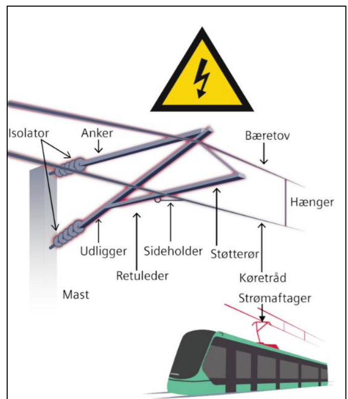
Principskitse
