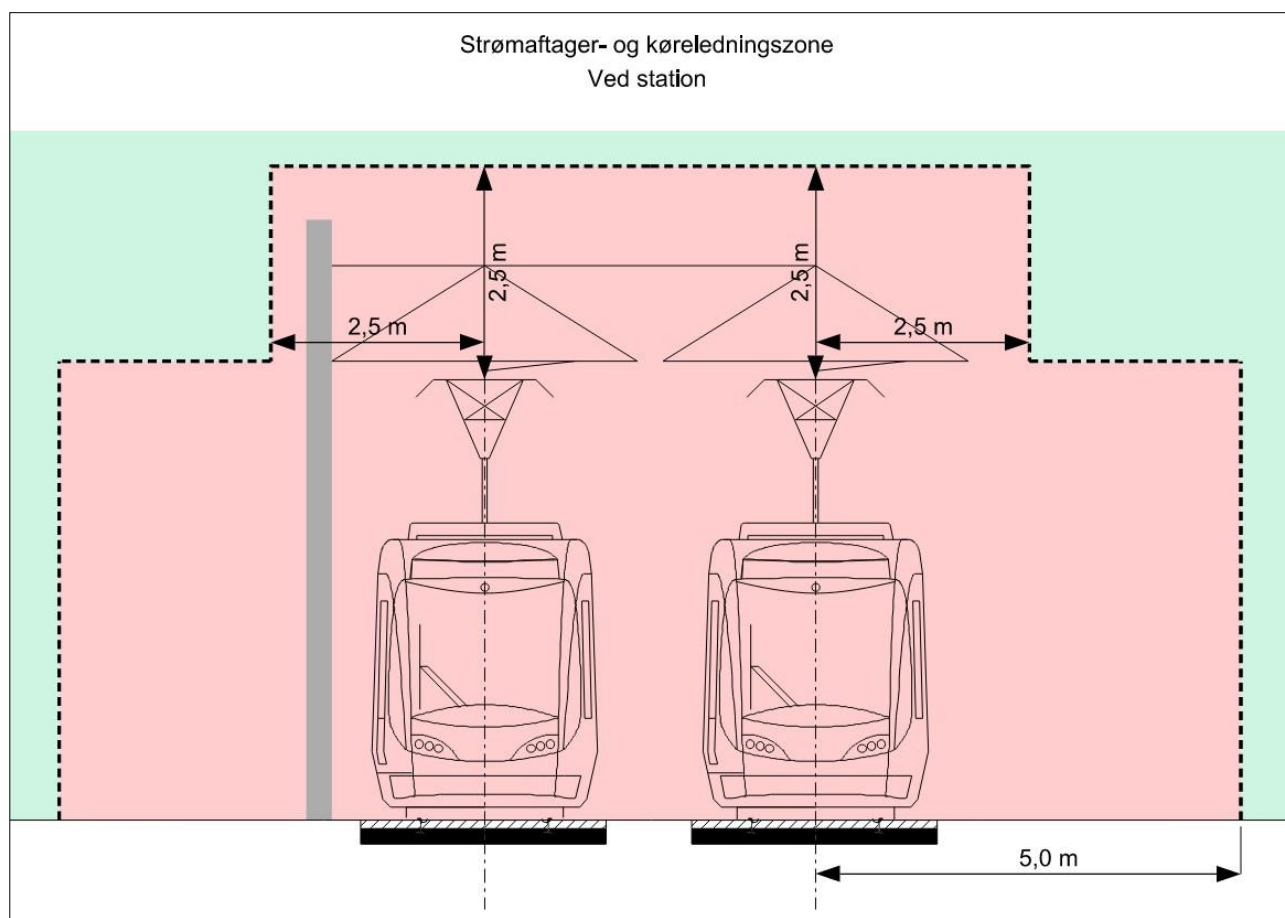
Principskitse
