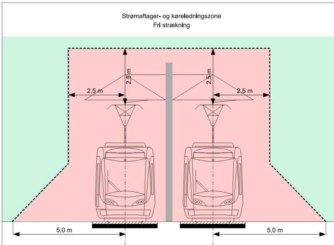
Principskitse
